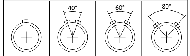
定位销图例
